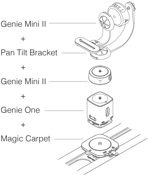
Genie One 3-Axis - Custom Build
